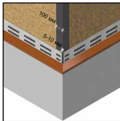
Рис. 8 Монтаж стартовой полосы.
