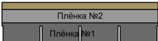
Рис. 10 Тыльная сторона фасадной плитки.
